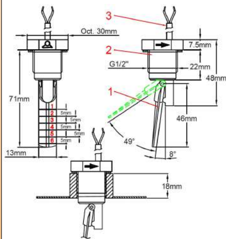
1: 柴叶 2: 主体 3: 电缆 R1S ( \frac{1}{2} " BSPP)
